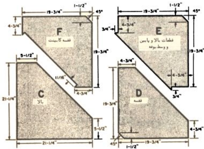
جزئیات قفسه‌ها و طبقات بوفه
