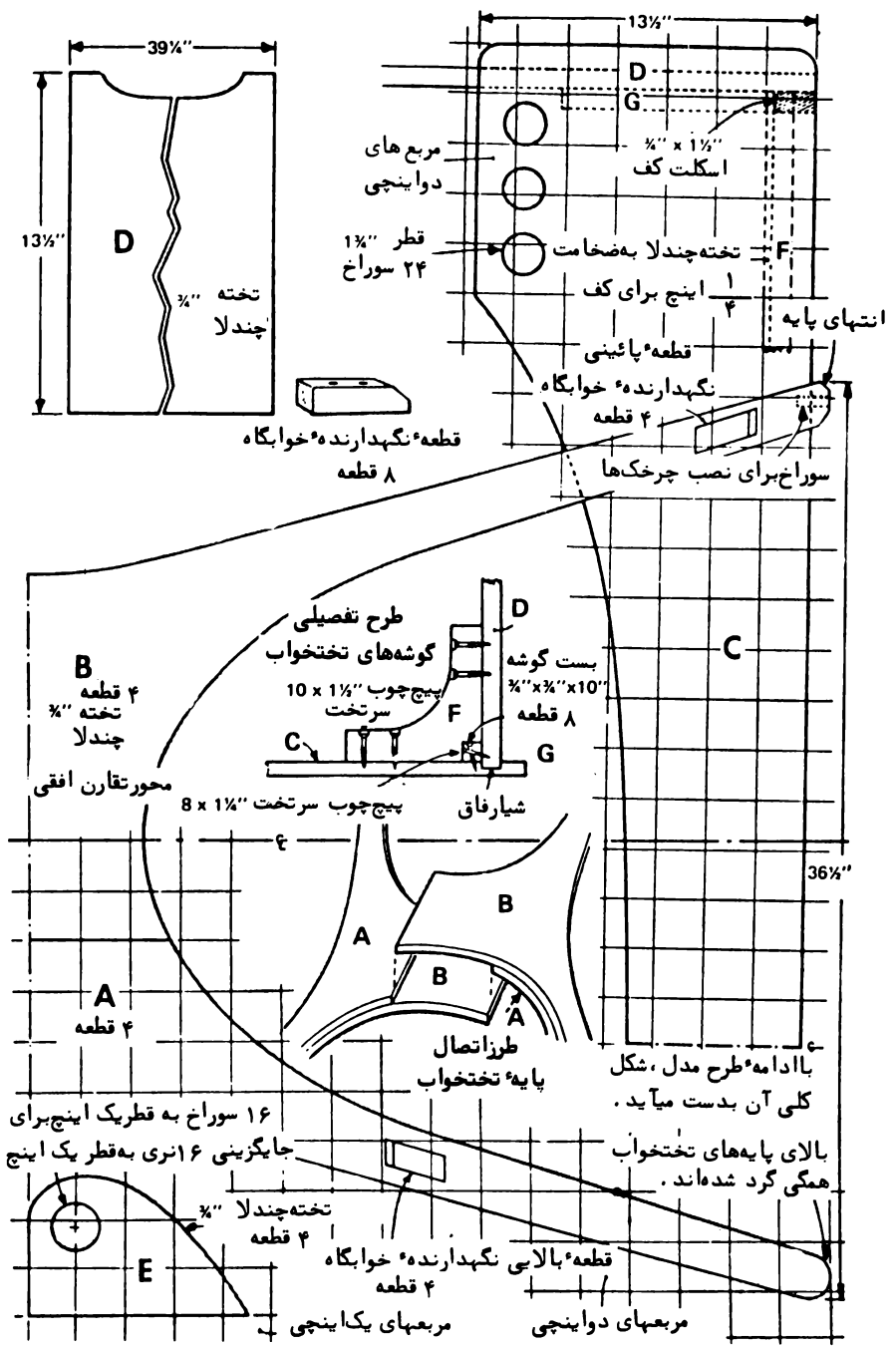
جزئیات کلی طرح تختخواب
