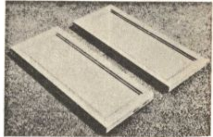
شکل ۷ - در شکل درهای تکمیل شده بوفه را مشاهده مینمائید که بعداً "به‌وسیله" لولای چاقویی به بدنه بوفه متصل خواهند شد.
