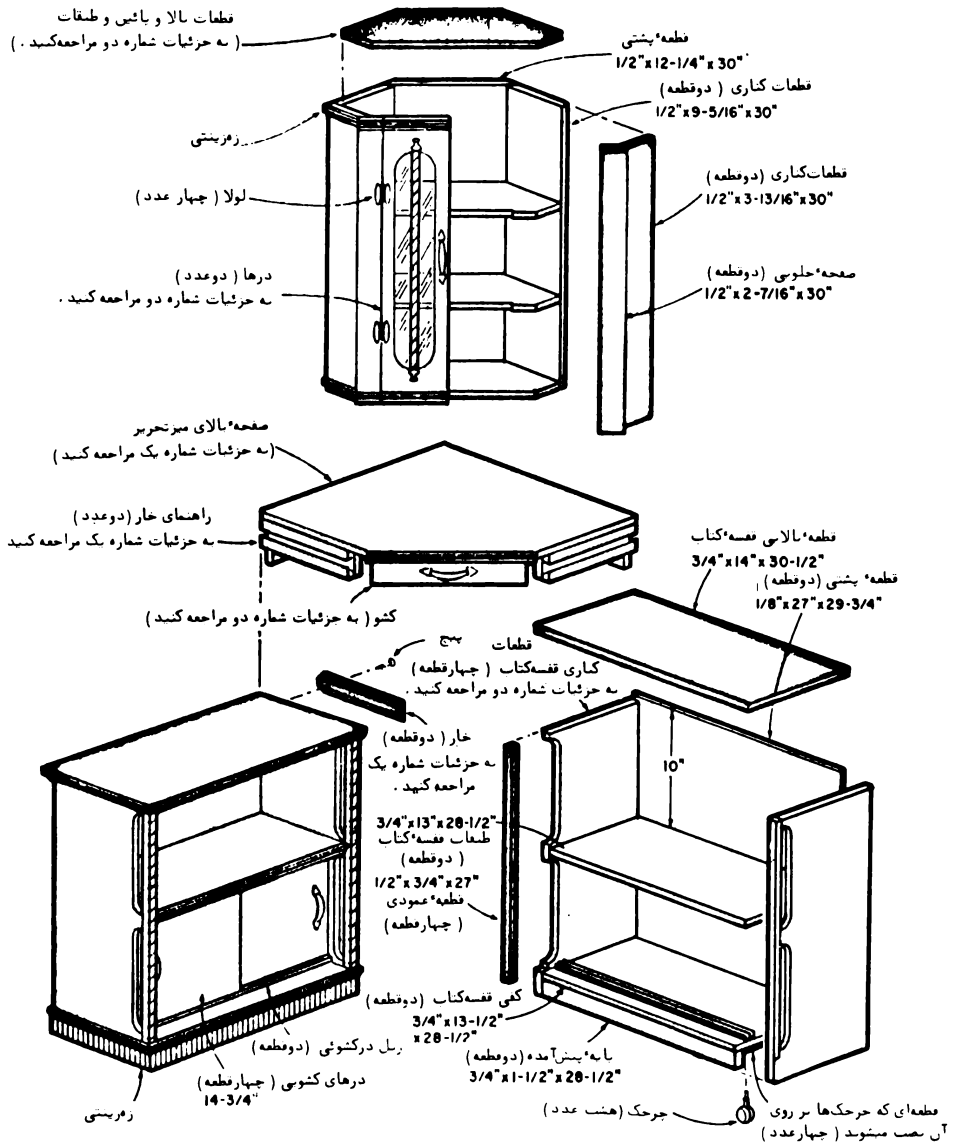
نمای گسترده کلیه قطعات طرح میز تحریر
