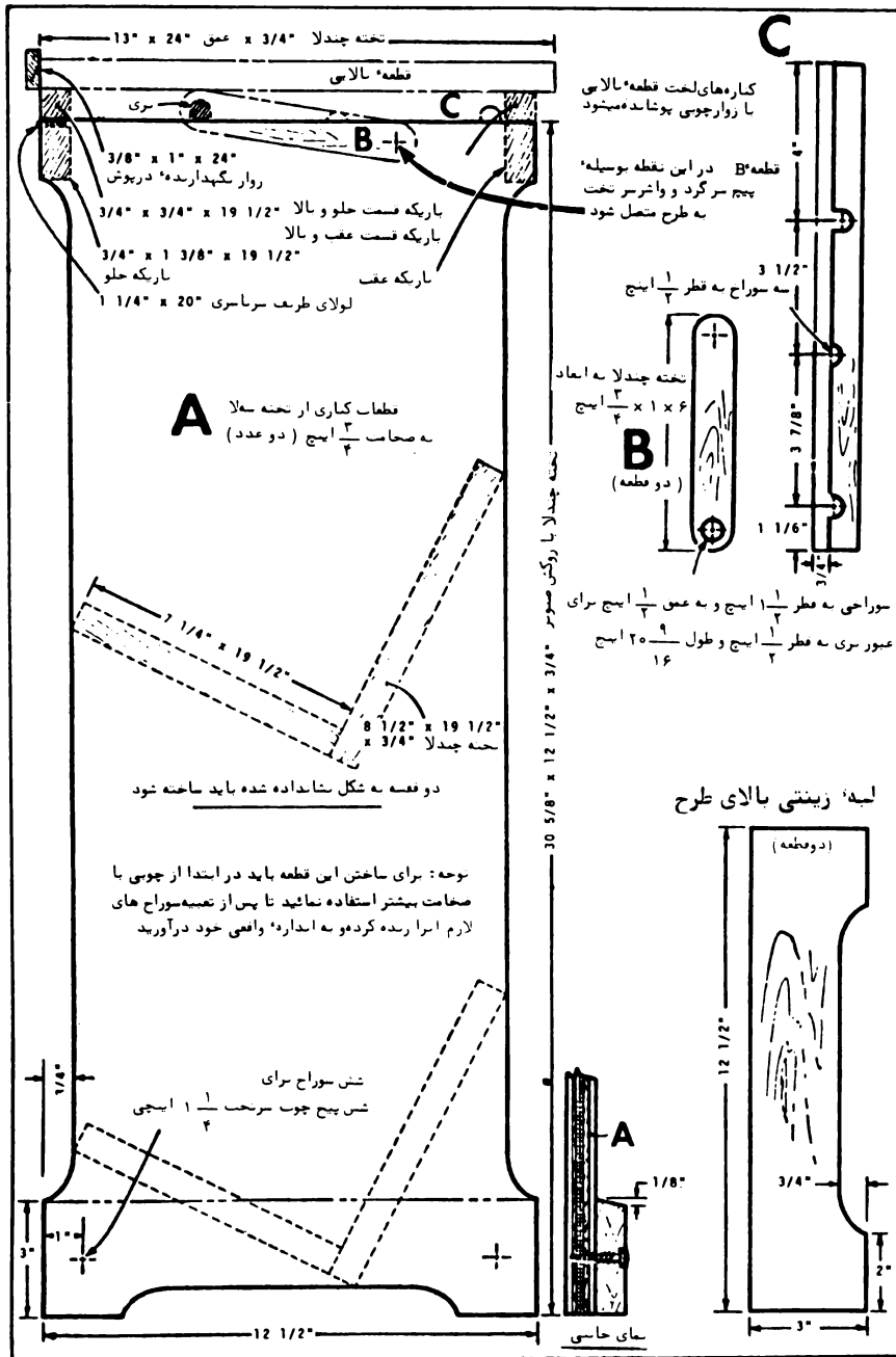
جزئیات کلی طرح
