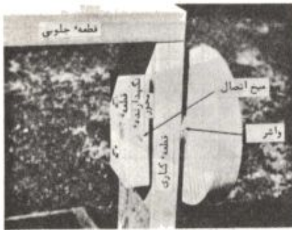
شکل ۵ - در شکل مجموعه قطعات مربوط به چرخ نشان داده شده است. در اینجا نحوه قفل شدن محور نری درقطعه نگهدارنده آن بوسیله میخ اتصال نشان داده شده است.
