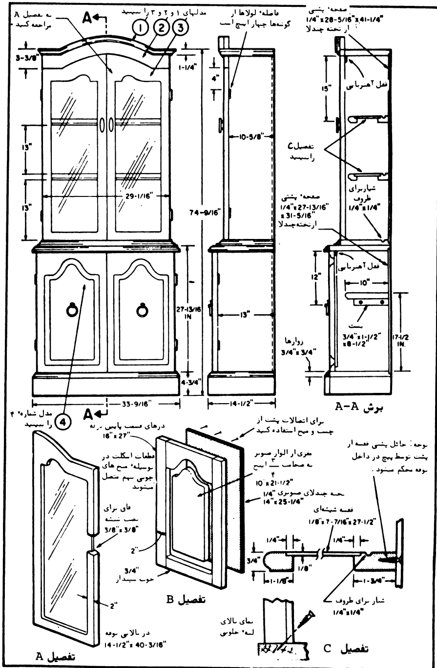
جزئیات طرح بوفه
