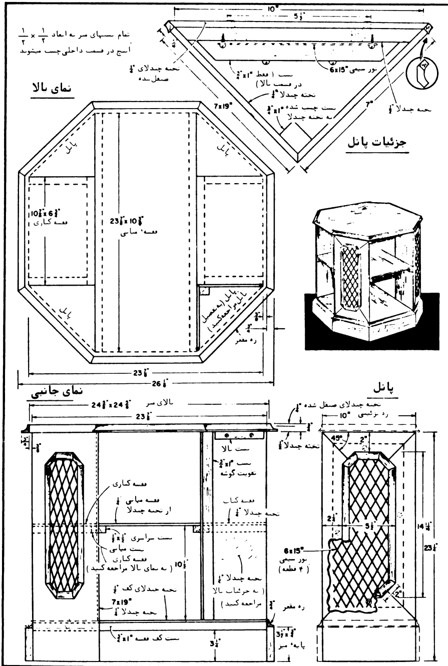
جزئیات و نماهای جانبی و بالای طرح
