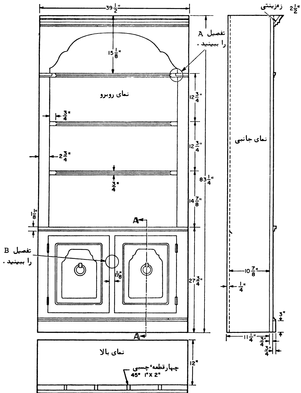
نمای روبرو و بالا و پائین طرح
