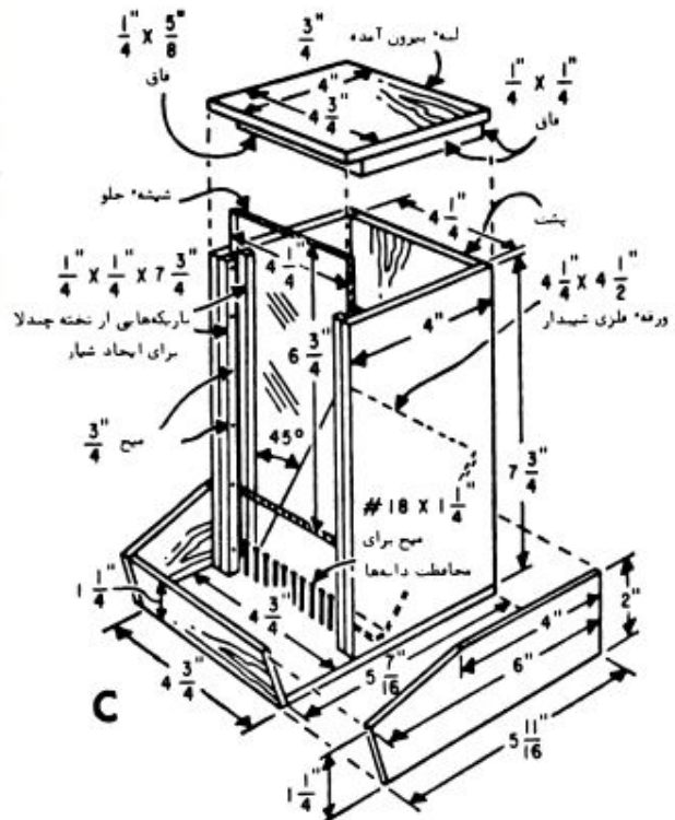
جزئیات انبار دانه که دو عدد از آن مورد احتیاج است
