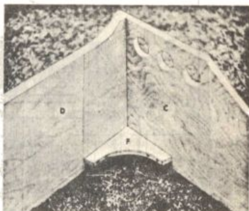
شکل ۴ - محل قرار گرفتن بست گوشه (F) برای محکم کردن قطعات کناری C و D و همچنین نگهداشتن کفی تختخواب روی قاب آن نشان داده شده است.
