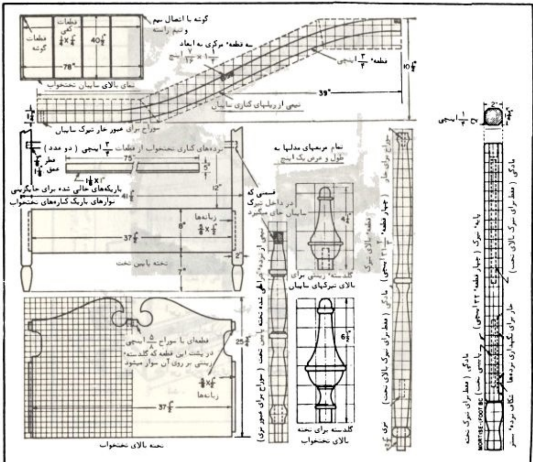
نمای گسترده‌ای از کلیه قطعات طرح
