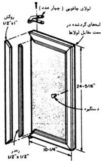
جزئیات درها
