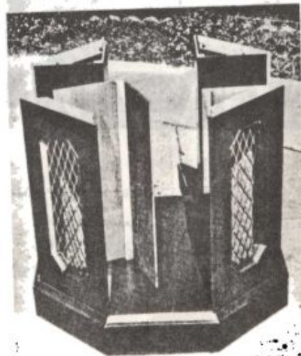
شکلهای ۸ و ۹ و ۱۰- قبل از خشک شدن چسب برای تثبیت زه‌های کناره، وجوه از چسب نواری استفاده نمایید. در اینجا همچنین نحوه اتصال زوارهای کناره، جای نصب توری سیمی نشان داده شده است. اگر بخواهید بستهای سرتاسری طرح را حذف کنید باید از اتصال فاق و زبانه استفاده کنید.
