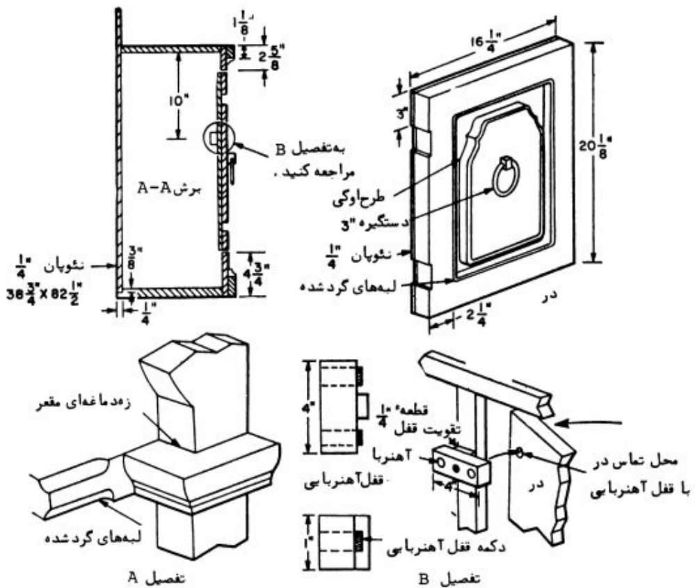
تفصیل در و قفل آهنربایی
