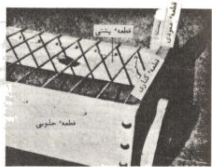
شکل ۶ - طناب کشی کردن زیر نیمکت ازین قطعات جلو و عقب شروع میشود. به نحوه عبور طناب از سوراخهای قطعات جلو و عقب دقت کنید.
