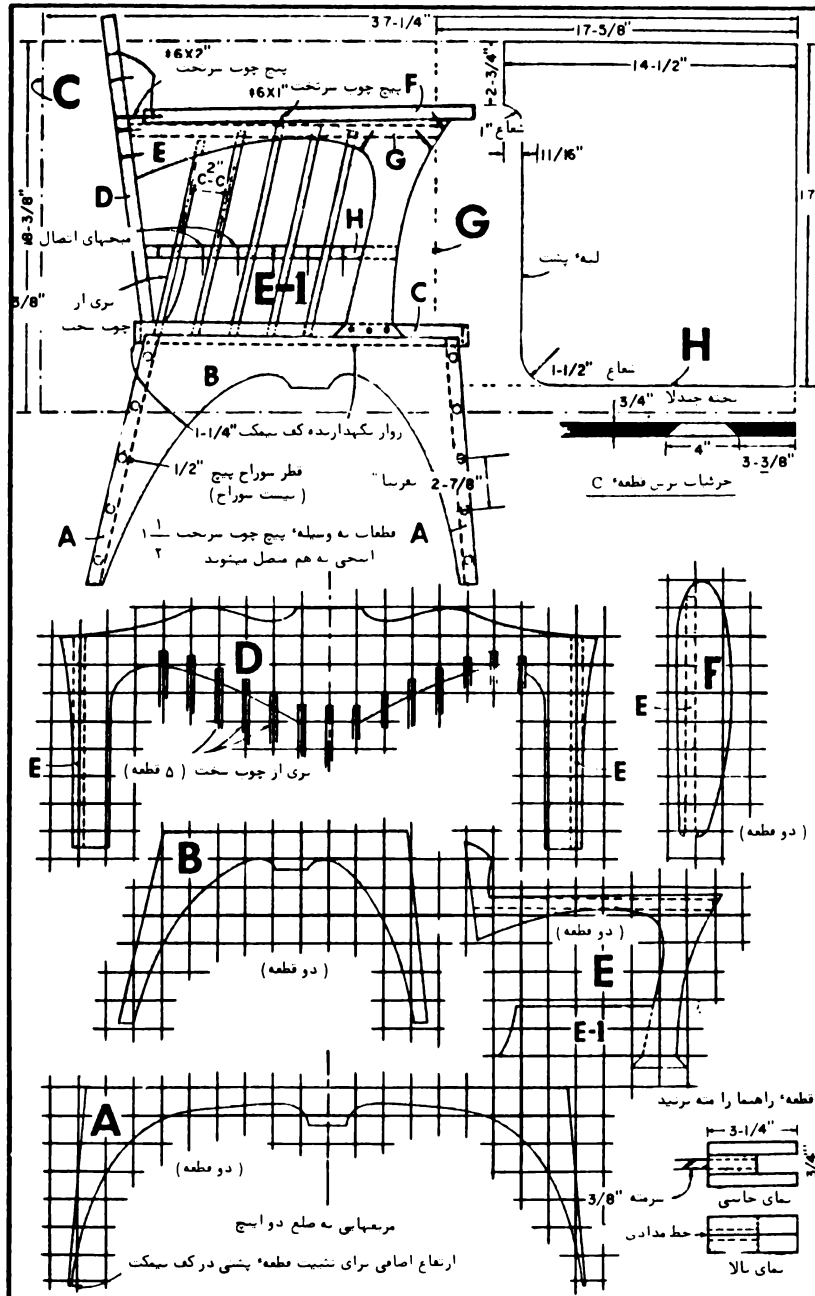
جزئیات و مدل‌های قطعات مختلف نیمکت و میز تحریر
