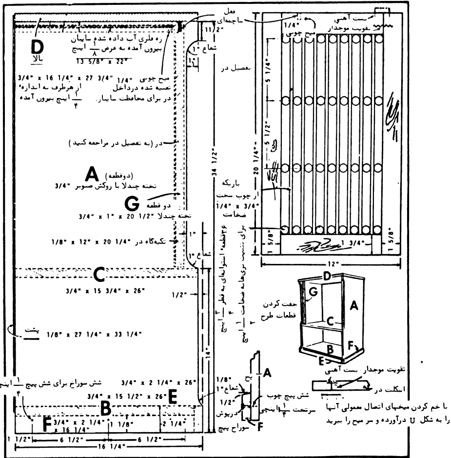
جزئیات طرح کابینت
