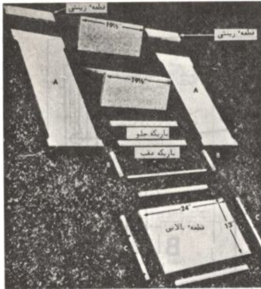
شکل ۱ - کلیه قطعات لازم برای ساخت این طرح در شکل نشان داده شده است. برای جفت کردن قطعات به حرز نشات طرح مراجعه کنید.
