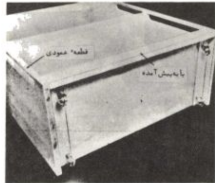
شکل ۲ - قسمت زیر قفسه کتاب پس از نصب چرخکها و پایه پیش آمده و قطعات عمودی نشان داده شده است. برای نصب چرخکها از یک قطعه نخته چندلا به ضخامت \frac{1}{4} اینچ استفاده شده است.
