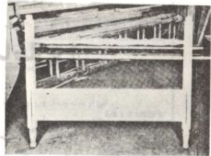
شکل ۲ - تخته پایین تخت قبل از نصب قسمت‌های بالایی تیرک‌ها در شکل دیده می‌شود. نرده‌ها در دو قسمت تهیه و نصب می‌شوند.
