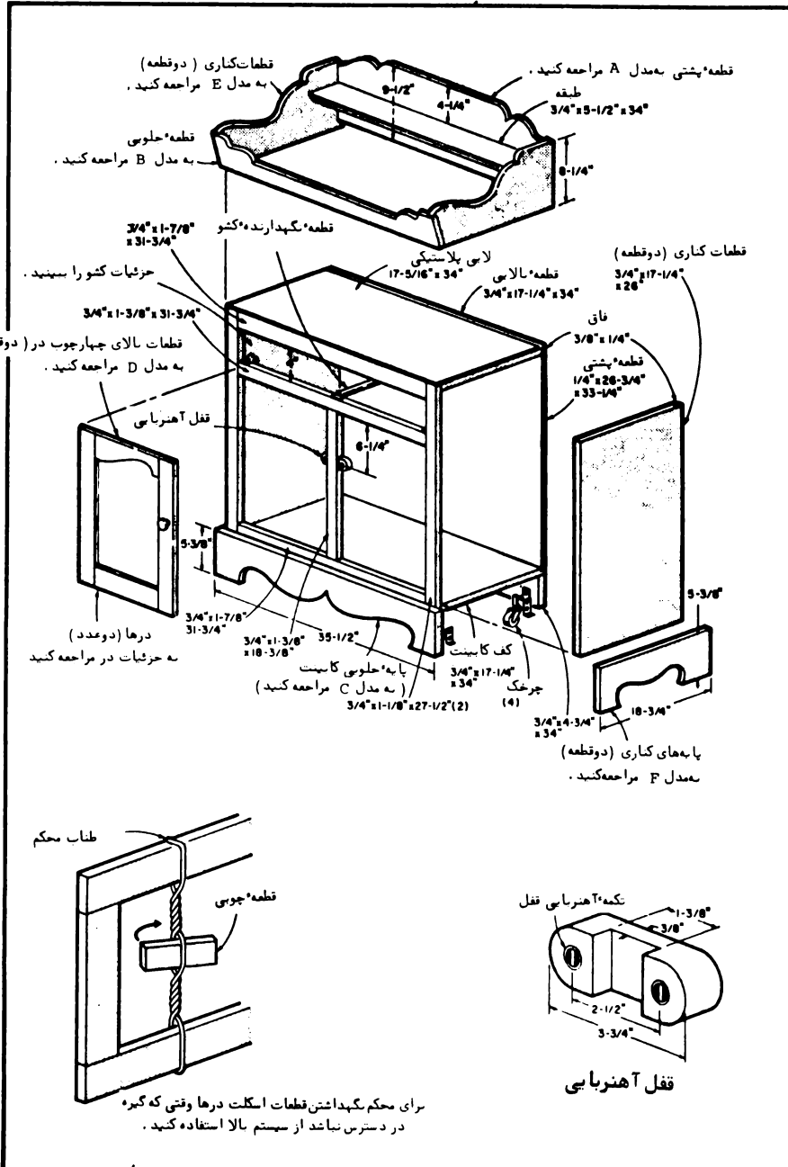
حزبیت کلی طرح و قفل آهنربایی آن
