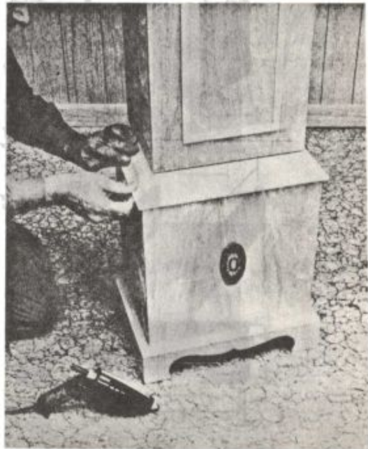
شکل ۳ - ساده‌ترین راه برای نصب زه مقعر استفاده از چسب گرم است که در مدت یکساعت محکم می‌شود.
