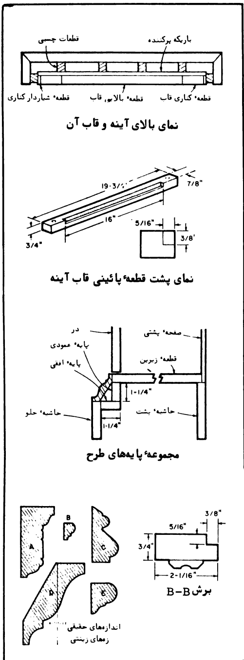
جزئیات شماره یک
