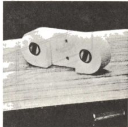
شکل ۶ - قطعات آهنربا را در سوراخهای قطعه نشان داده شده در شکل جای داده و آنرا به قطعه عمودی اسکلت جلوی طرح پیچ کنید.
