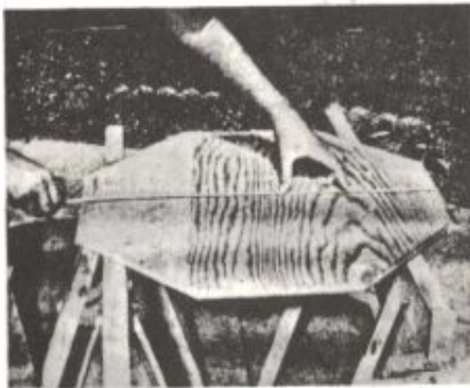
شکل ۳ - اگر در نظر دارید سطح میز به شکل هشت ضلعی منظم باشد قبل از نصب، اندازه‌های آن، بخصوص فاصله بین دو ضلع روبرو را بدقت اندازه‌گیری کنید.
