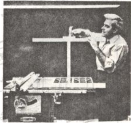
شکل ۳ - برای اتصال قطعات اسکلت قسمت جلوی کابینت از چکش و یک تکه چوب بنحوی که در شکل نشان داده شده استفاده کنید .
