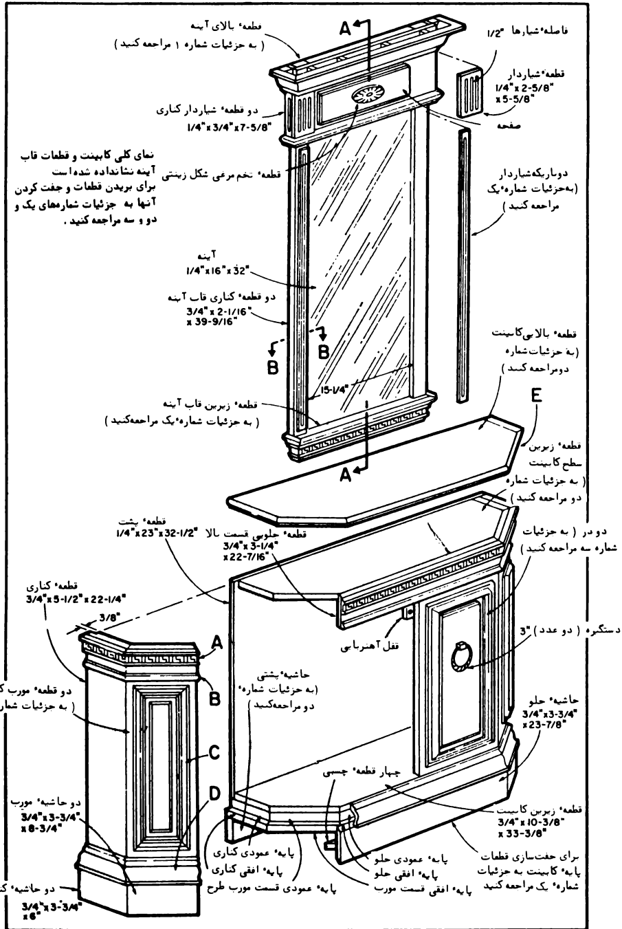
جزئیات کلی طرح
