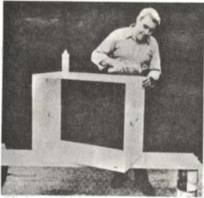
شکل ۲ - اسکلت قسمت جلوی کابینت را بدقت سر هم کرده و برای استحکام بیشتر آن از میخهای چوبی استفاده نمائید .
