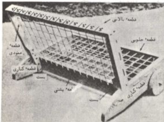
شکل ۷ - نمایی از قسمت عقب طرح کامل شده نیمکت که در آن باید به نوع بافت طناب توجه کرد. مثلاً "باید توجه داشت که طنابهای بافته شده پشت و زیر نیمکت هر دو از قطعه پستی از یک سوراخ رد میشوند.
