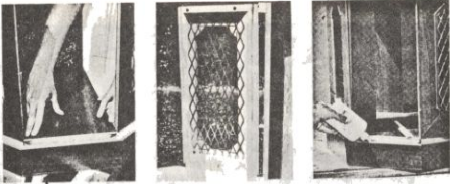
شکلهای ۵ و ۶ و ۷- قبل از جفت کردن قطعات طرح تورسیمی را با پیچ درجای خود محکم کنید و سپس قطعات را با چسب سفید بهم متصل نمایید.
