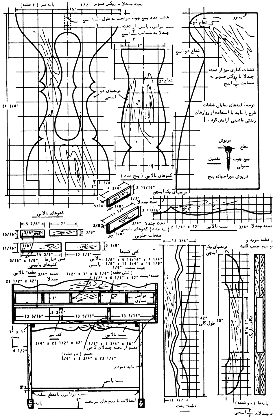
جزئیات و ابعاد مختلف میز تحریر
