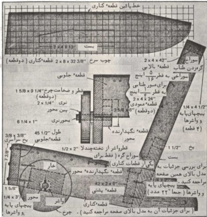
جزئیات طرح نیمکت
