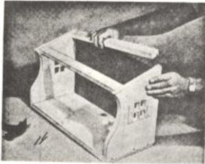
شکل ۱ - شاه تیر عقب را که لبه‌های آن گرد شده طوری نصب کنید که صفحه عقبی طرح در شمار آن جای گیرد.
