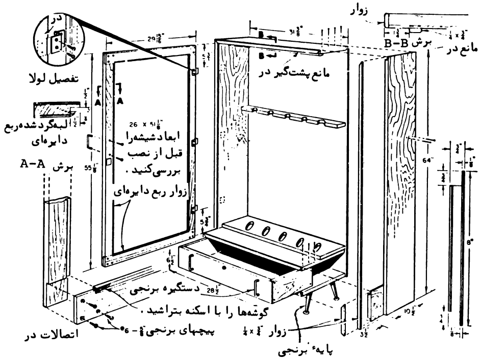
جزئیات قطعات کابینت
