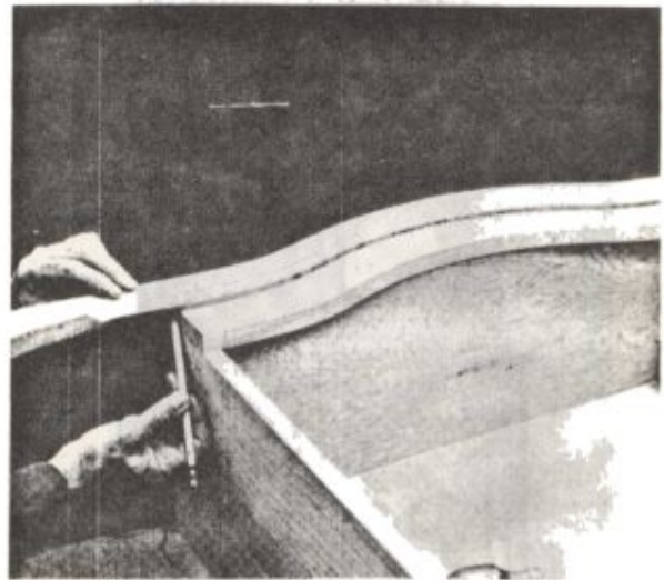
شکل ۴ - قبل از بریدن قطعه شکل داده شده آنرا به نحوی که در شکل نشان داده شده دقیقاً اندازه گیری کنید .
