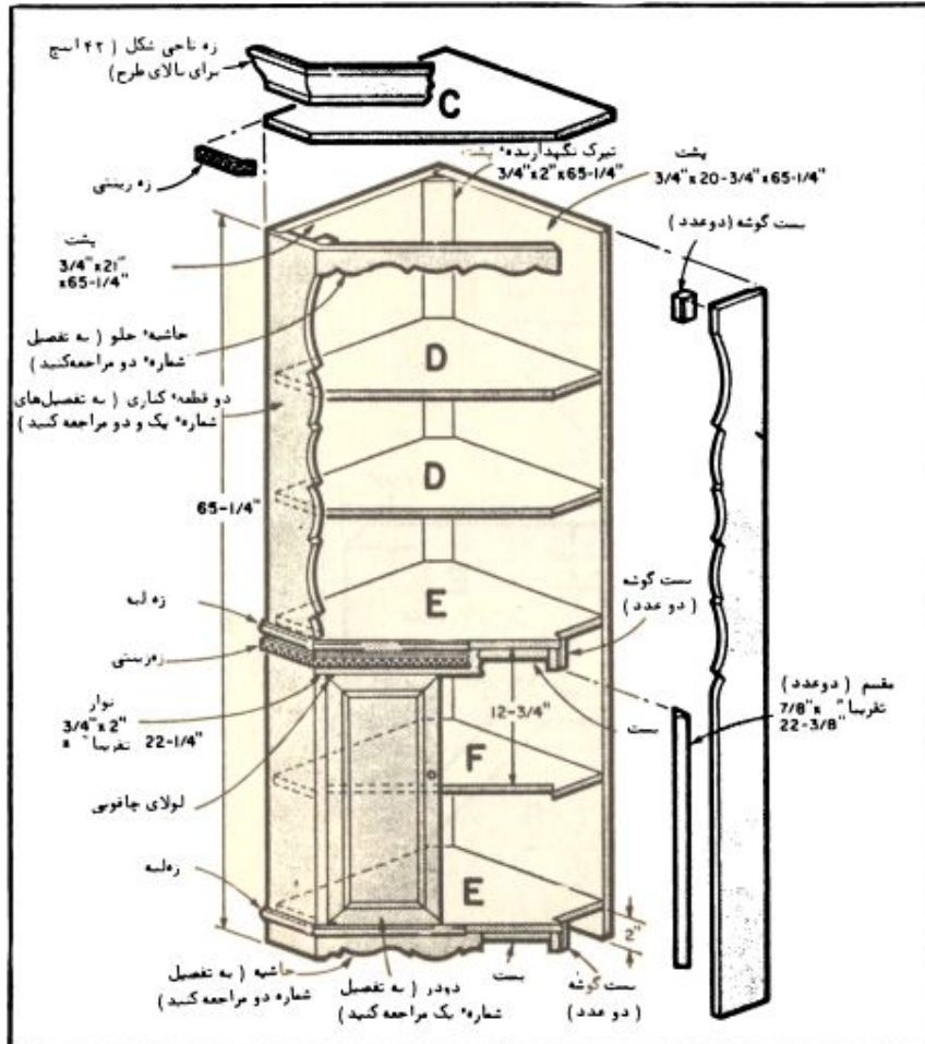
جزئیات طرح بوفه چوبی
