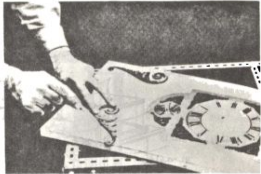
شکل ۲ - جای قرار گرفتن کنده‌کاریها را بر روی صفحه جلویی طبقه بالای ساعت علامتگذاری نموده و سپس ببرید.
