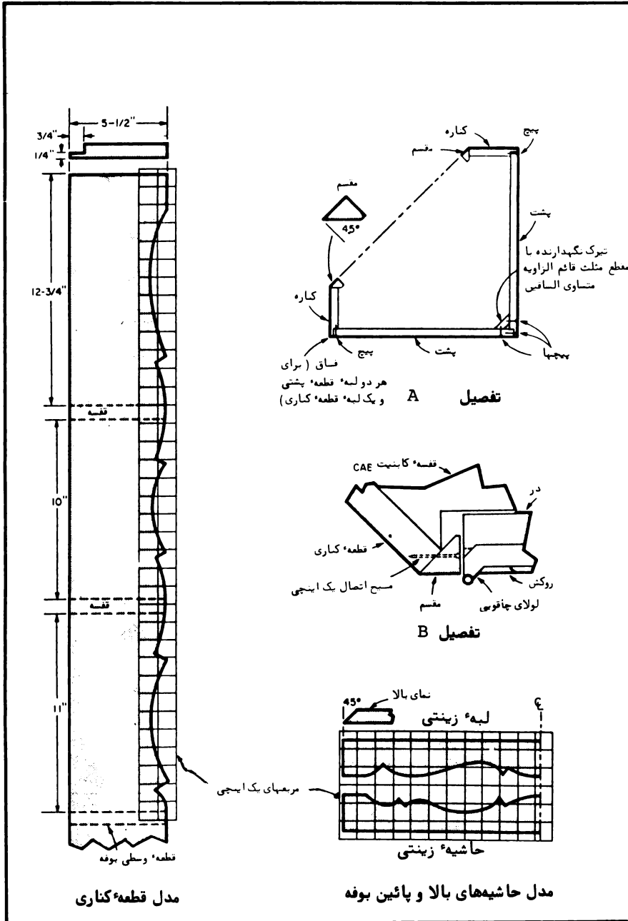
تفصیل شماره دو
