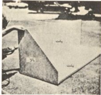
شکل ۲ - برای متصل کردن قطعات بوسیله چسب و میخ از قسمت پشت شروع کنید و سپس قسمت بالای بوفه راه وسیله پیچ به قطعات پشتی متصل سازید .
