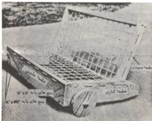
شکل ۸ - سه چهارم از نمای حلوی طرح کامل شده در شکل دیده میشود. نحوه عبور طناب از قطعات حلوی و کناری و همچنین محل نصب چرخ توجه کنید.
