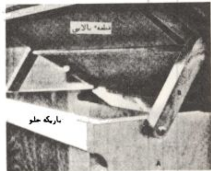
شکل ۴ - نمای دیگری از قطعه B که نگهدارنده قطعه بالایی است در اینجا نشان داده شده است. توجه کنید که قطعات چگونه بدقت باید بهم جفت شوند. با خارج کردن ضام قطعه B میتوان قطعه C را به عنوان در برای خاکناسی استفاده نمود.
