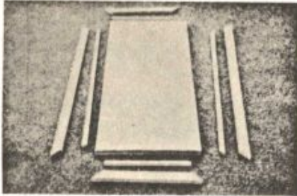
شکل ۶ - زوارهای دور در را بوسیله پیچ‌های یک‌اینچی از قسمت پشت و زه زینتی را بوسیله چسب به در بوفه چسبانید.
