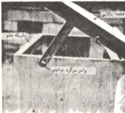
شکل ۳ - ضام قطعه B که برای نگهداری قطعه C در زوایای مناسب تعبیه شده باید در یکی از سه نمدایره موجود در قطعه C قرار گیرد.
